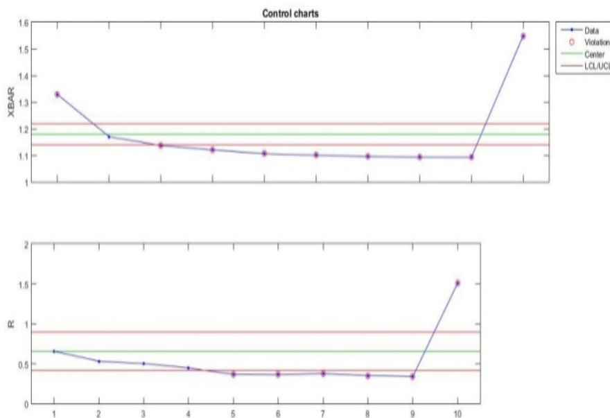
شکل ۲. نمودار کنترلی X و R شاخص DPI خروجی نرم افزار Matlab
